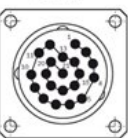
Ansicht Gerüststecker M23, 21-polig am Encoder, Parallel
