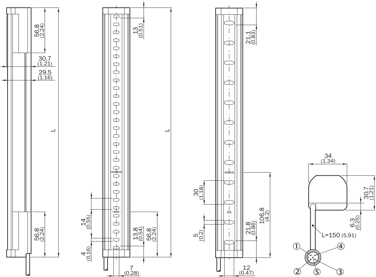
Габаритный чертёж (Размеры, мм)
