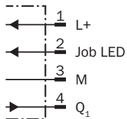
Empfänger
