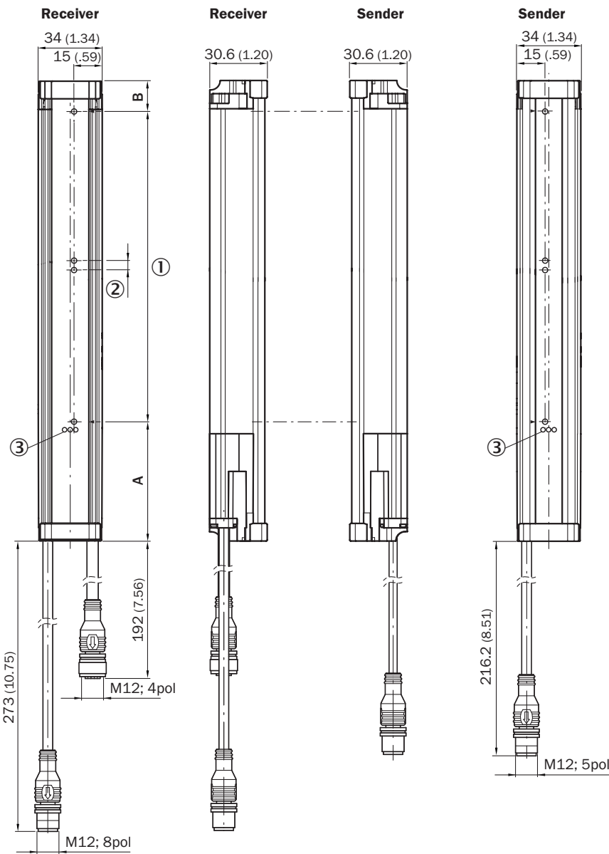
Габаритный чертеж
