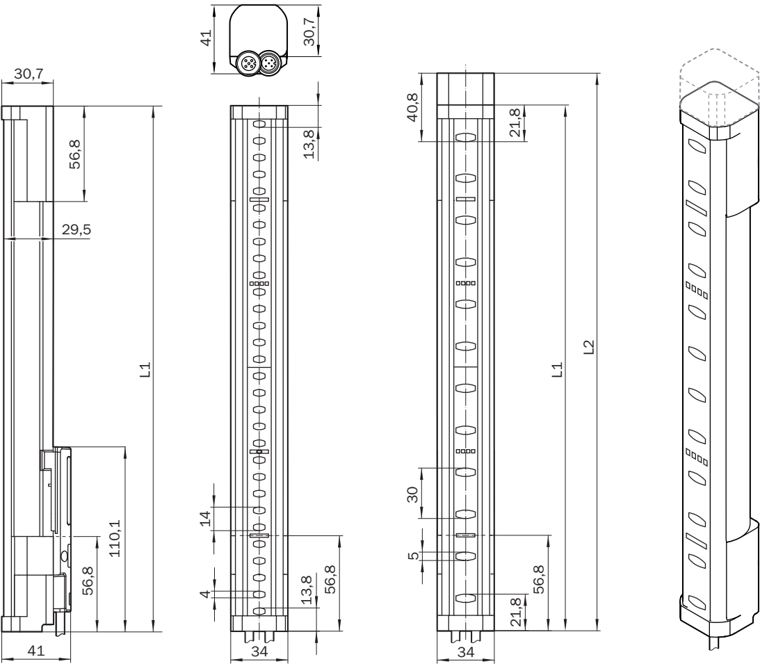
Maßzeichnung (Maße in mm)
