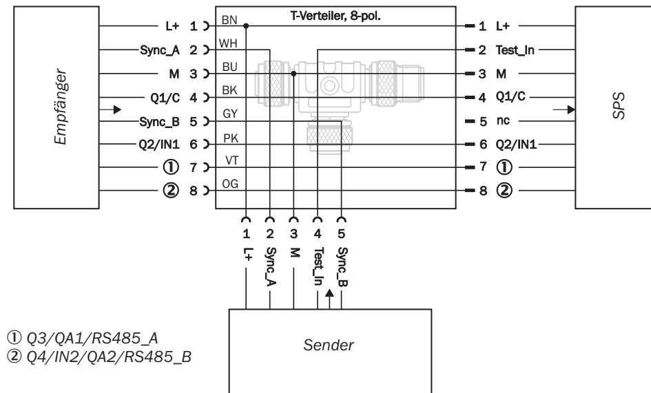
Anschlussschema T-Verteiler
