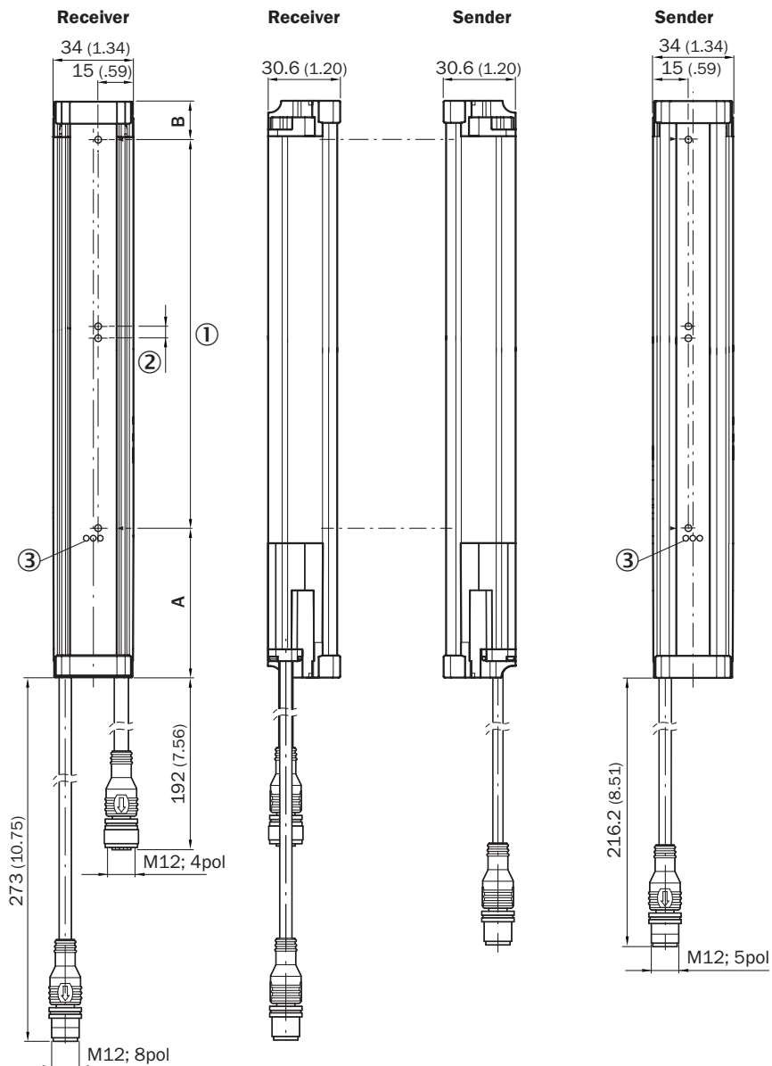
Rysunek wymiarowy
