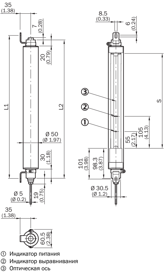
Габаритный чертеж (Размеры, мм)
