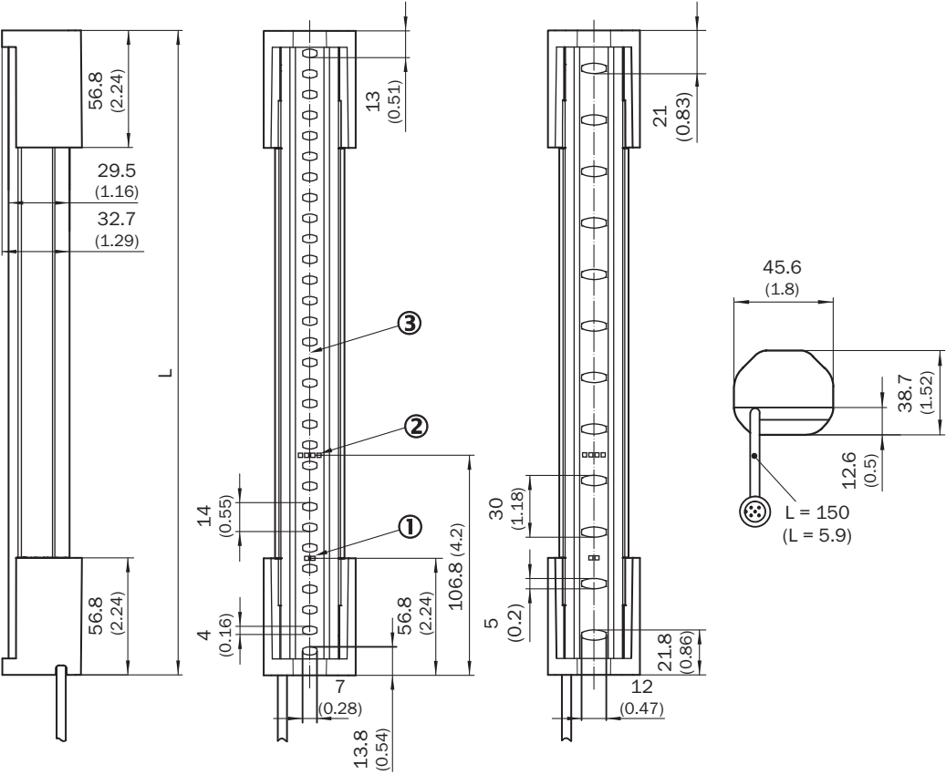
Габаритный чертеж (Размеры, мм)
