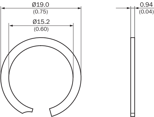
Волновая пружина
