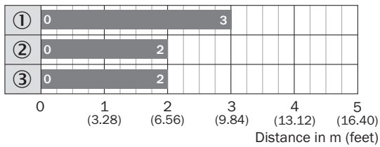
Wykres zasięgu wykrywania (MDO 5 mm)
