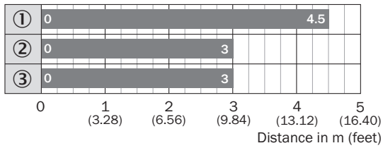
Wykres zasięgu wykrywania (MDO 10 mm)
