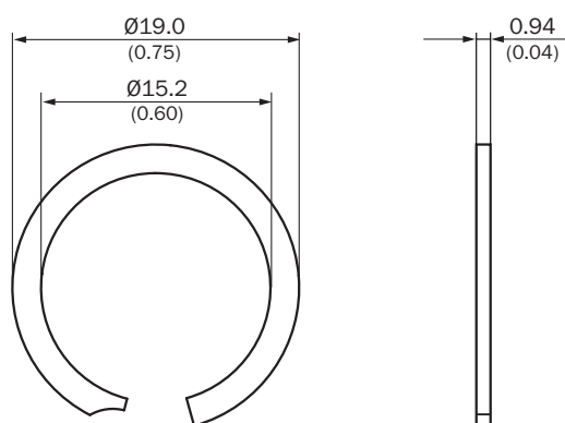
Волновая пружина
