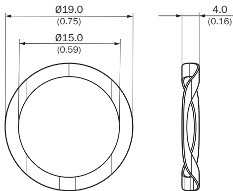
Sprężyna wałka
