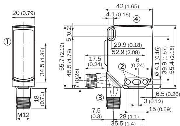
Rysunek wymiarowy (Wymiary w mm)
