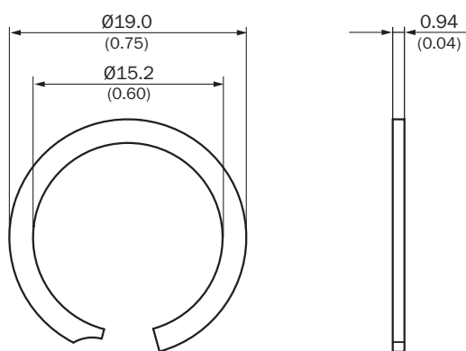
Sprężyna wałka
