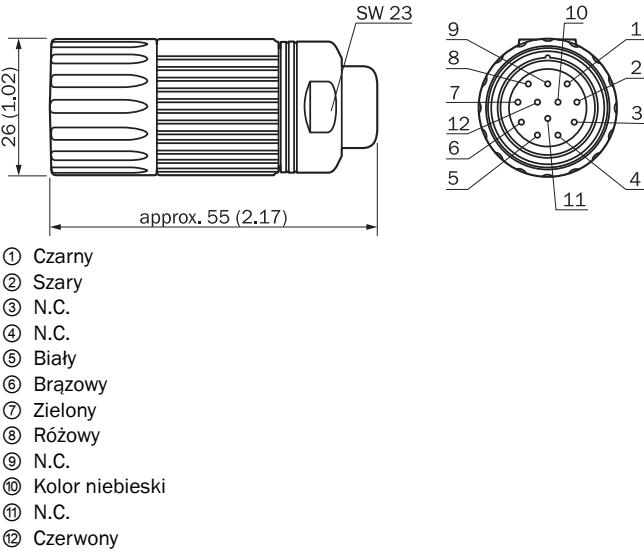
Rysunek wymiarowy (Wymiary w mm)
