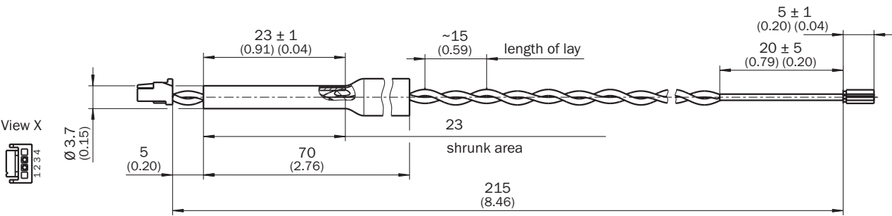
Rysunek wymiarowy (Wymiary w mm)
