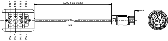
Rysunek wymiarowy (Wymiary w mm)
