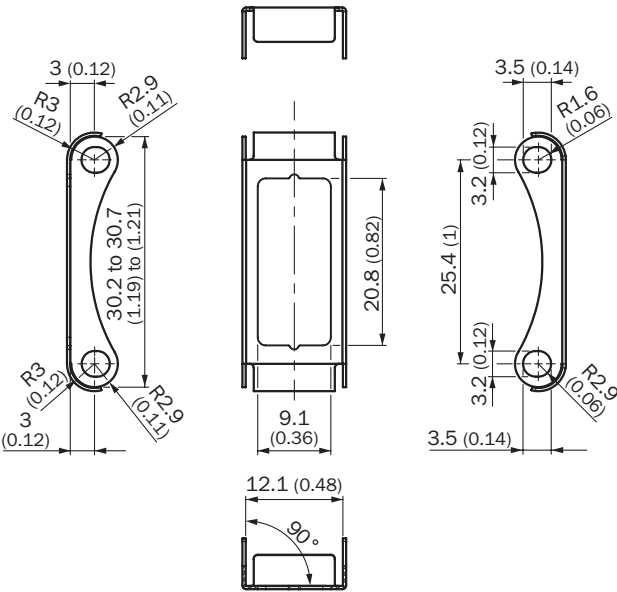
Rysunek wymiarowy (Wymiary w mm)
