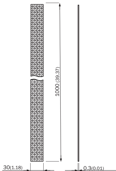
Rysunek wymiarowy (Wymiary w mm)
