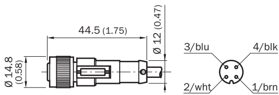
Rysunek wymiarowy (Wymiary w mm)
