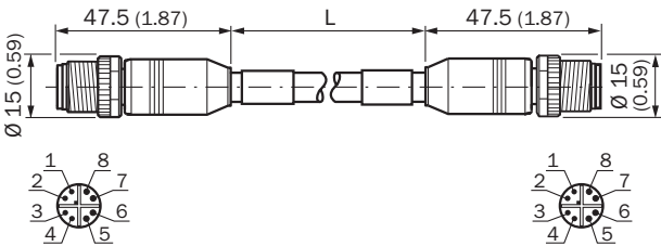
Rysunek wymiarowy (Wymiary w mm)
