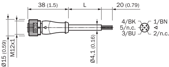
Rysunek wymiarowy (Wymiary w mm)
