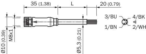
Rysunek wymiarowy (Wymiary w mm)
