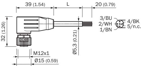
Rysunek wymiarowy (Wymiary w mm)
