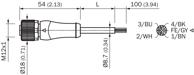
Rysunek wymiarowy (Wymiary w mm)
