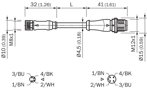
Rysunek wymiarowy (Wymiary w mm)
