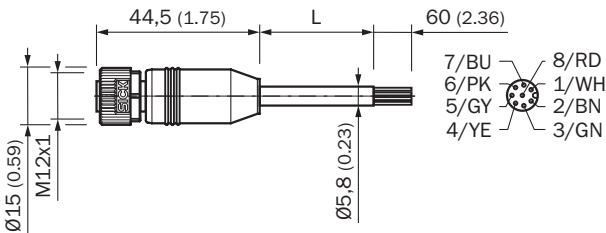
Габаритный чертёж (Размеры, мм)
