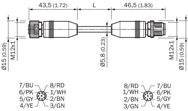
Rysunek wymiarowy (Wymiary w mm)
