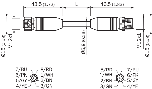
Rysunek wymiarowy (Wymiary w mm)
