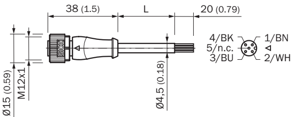
Габаритный чертёж (Размеры, мм)
