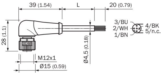
Габаритный чертёж (Размеры, мм)
