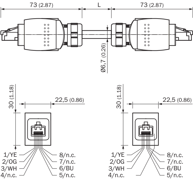
Rysunek wymiarowy (Wymiary w mm)
