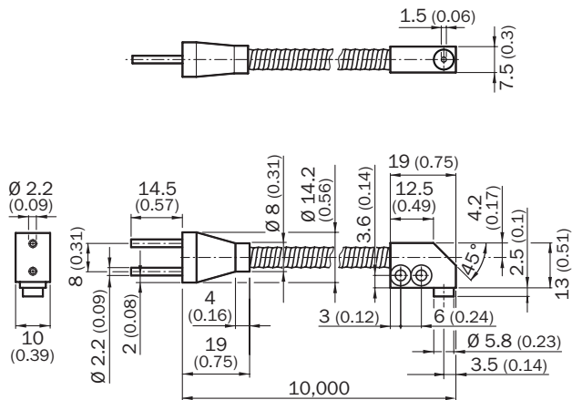
Rysunek wymiarowy (Wymiary w mm)
