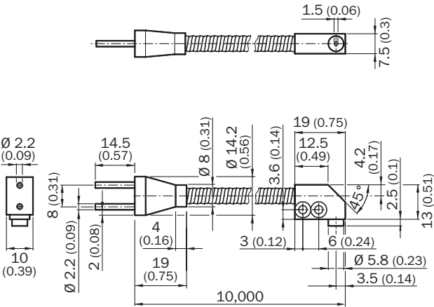
Габаритный чертеж (Размеры, мм)
