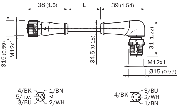
Rysunek wymiarowy (Wymiary w mm)
