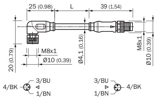
Rysunek wymiarowy (Wymiary w mm)
