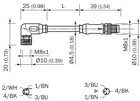
Rysunek wymiarowy (Wymiary w mm)
