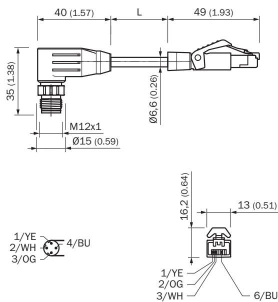
Rysunek wymiarowy (Wymiary w mm)
