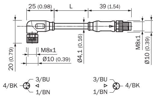
Rysunek wymiarowy (Wymiary w mm)
