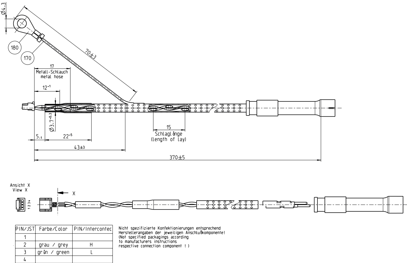
Rysunek wymiarowy (Wymiary w mm)
