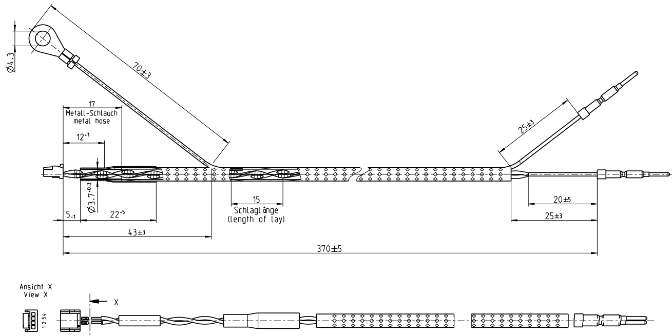
Rysunek wymiarowy (Wymiary w mm)
