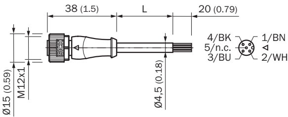
Габаритный чертеж (Размеры, мм)
