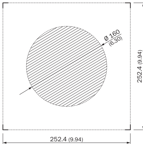
Rysunek wymiarowy (Wymiary w mm)
