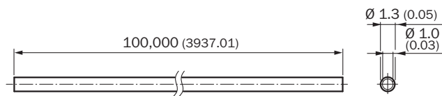
Rysunek wymiarowy (Wymiary w mm)
