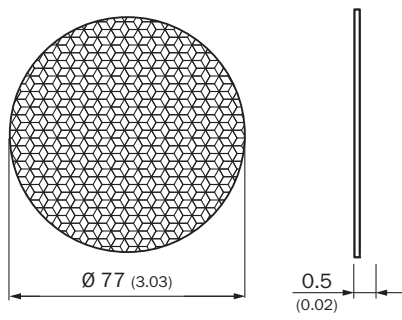
Rysunek wymiarowy (Wymiary w mm)
