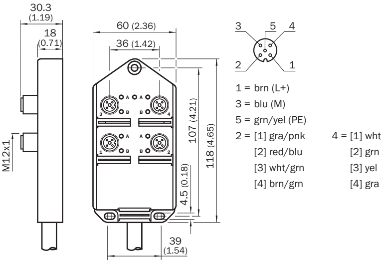
Rysunek wymiarowy (Wymiary w mm)
