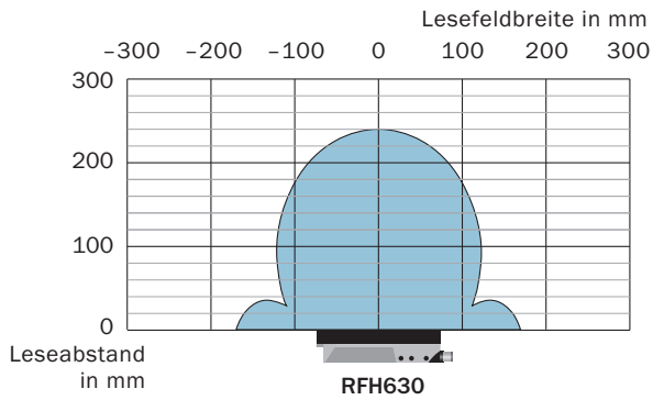
Lesefelddiagramm RFH63x
