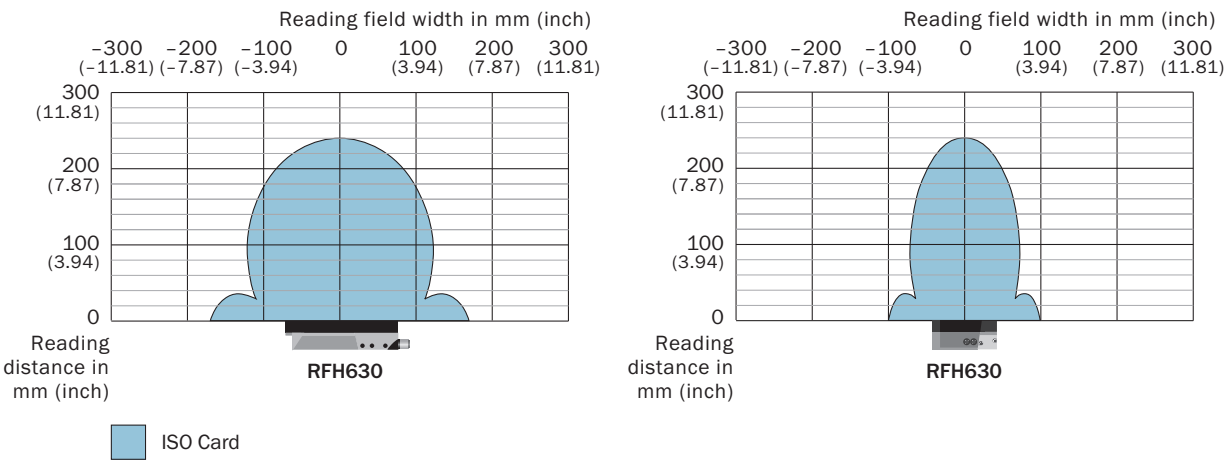
Диаграмма поля считывания RFH62x
