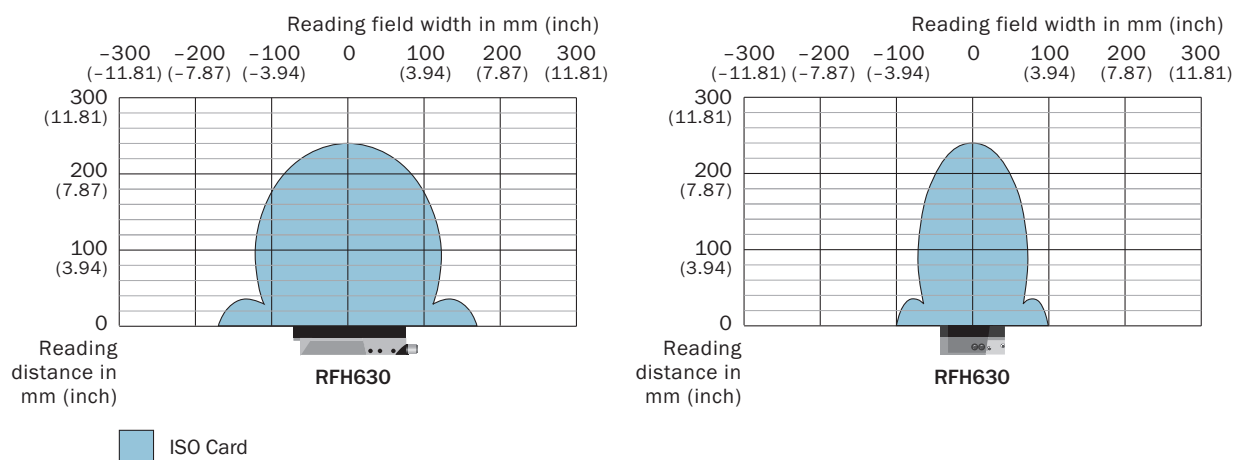
Wykres pola odczytu RFH62x
